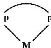
(کمپلکس کی لیت)
